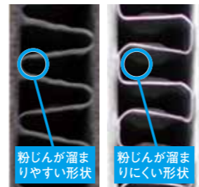
標準ラジエータ ワイドフィンラジエータ
