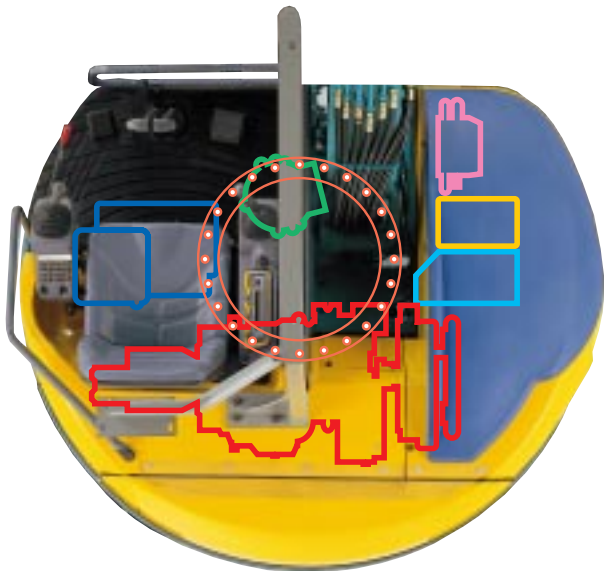
エンジン 燃料タンク バッテリー 旋回ベアリング 旋回モータ 油圧タンク コントロールバルブ
