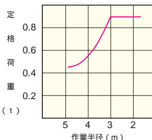
定格荷重線図及び荷重表 RX-503CR (標準アーム、0.22 バケット付)
